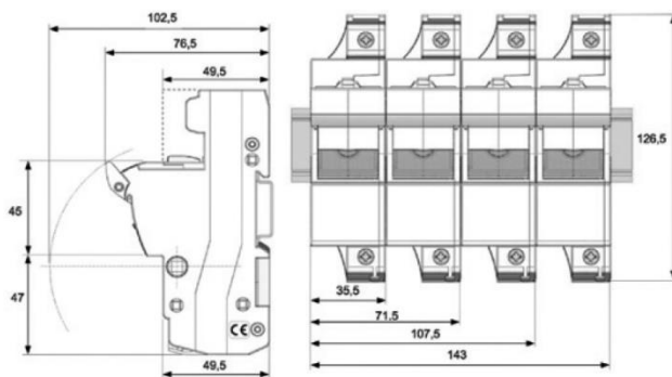
coupe-circuit 22x58
