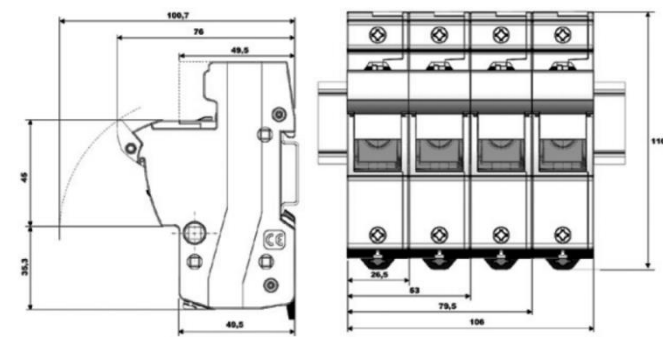
coupe-circuit 14x51
