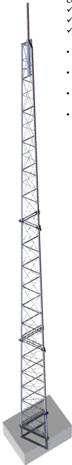
Pylône autoportant
